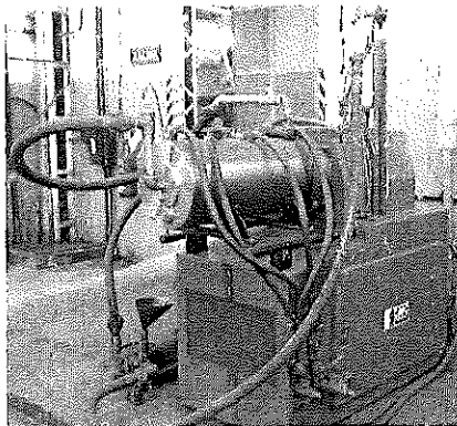
Molino de Arena 5: CMC Modelo 45 LITER MILL
