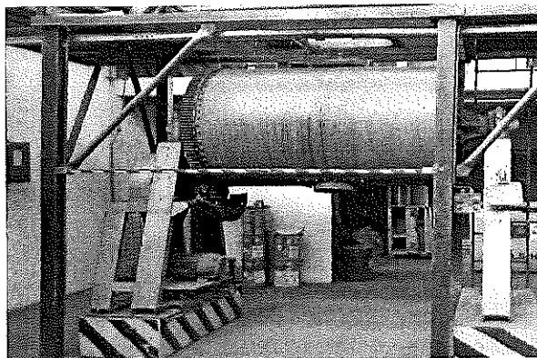
Molino de Bolas 2: Industria Argentina
